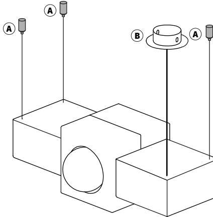
Decentralizer (3 pcs.)
